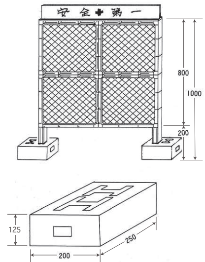
寸法図 (mm)
