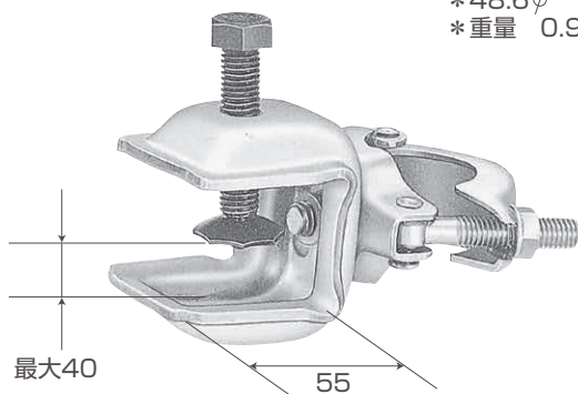
バイスクランプ(直自兼用)
