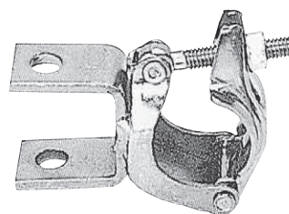
朝顔 蛙又クランプ
