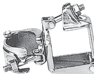
角丸クランプ(直交、自在)
