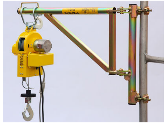
【吊りクランプ】
